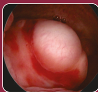
POLYP
